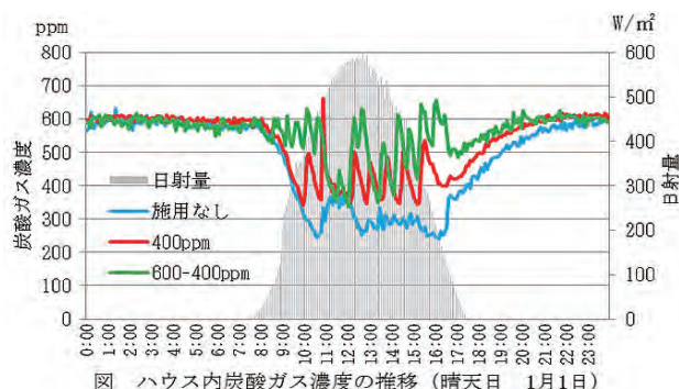
図 ハウス内炭酸ガス濃度の推移 (晴天日 1月1日)
