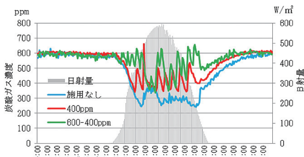
図 ハウス内炭酸ガス濃度の推移 (晴天日 1月1日)
